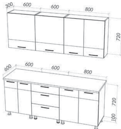
«Николь 14» 2140x2000x600 мм.
