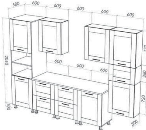
«Монако 6» 2140x3000x600 мм.
