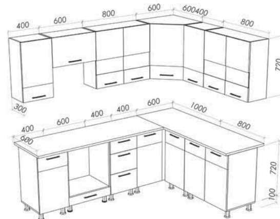
«Николь 16» 2140x2400x1800 мм.
