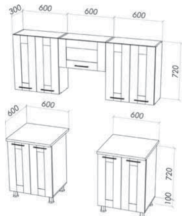
«Монако 12» 2140x2000x600 мм.
