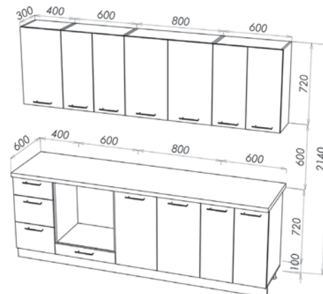
«Дельта 2.0» 2140x2400x600 мм.
