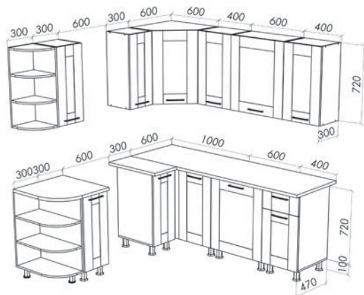
«Монако 3» 2140x3600x600 мм.
