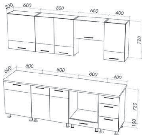
«Николь 6» 2140x2400x600 мм.
