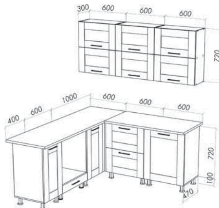
«Монако 5» 2140x2400x3800 мм.
