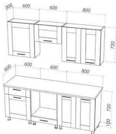
«Монако 12» 2140x2000x600 мм.
