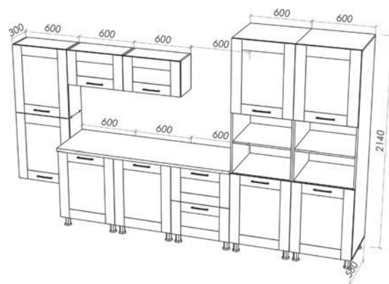
«Монако 3» 2140x3600x600 мм.
