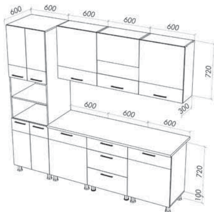
«Николь 3» 2140x2400x600 мм.
